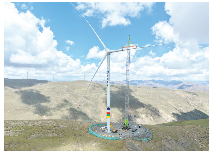
6月18日,中建二局承建的西藏华电琼结440MW风电基地一期150MW风电项目首台风机顺利在西藏山南市琼结县完成吊装,这座最高点海拔达5350米的超高海拔山地风电工程迎来施工关键节点。 新华社发
