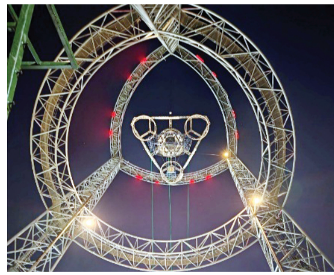
“逐日工程”空间太阳能电站地面验证系统(4月16日摄)。新华社发
