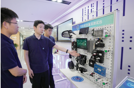
国家计算机病毒应急处理中心汽车安全漏洞测试台。记者 孙震 赵建伟 摄
