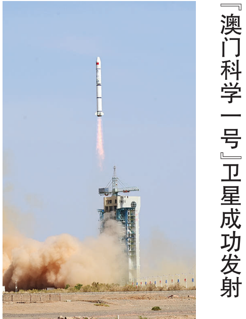
5月21日16时,我国在酒泉卫星发射中心采用长征二号丙运载火箭,成功发射首颗内地与澳门合作研制的空间科学卫星“澳门科学一号”。
