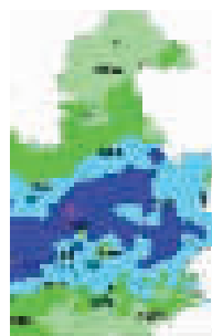
28日10时-16时降雨量
